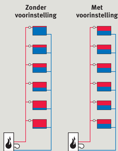
Waterverdeling in de verwarmingselementen na een nachtverlagingsperiode, waarbij alle thermostaatventielen zijn geopend. De rechter installatie heeft vooringestelde afsluiters, de linker niet.
